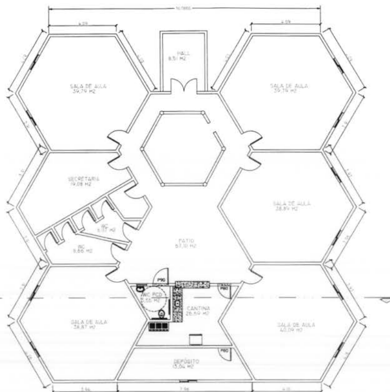
PLANTA BAIXA esc 1:150
