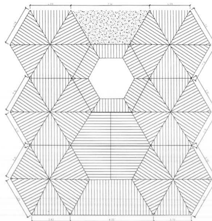
PLANTA DE COBERTURA esc 1:150
